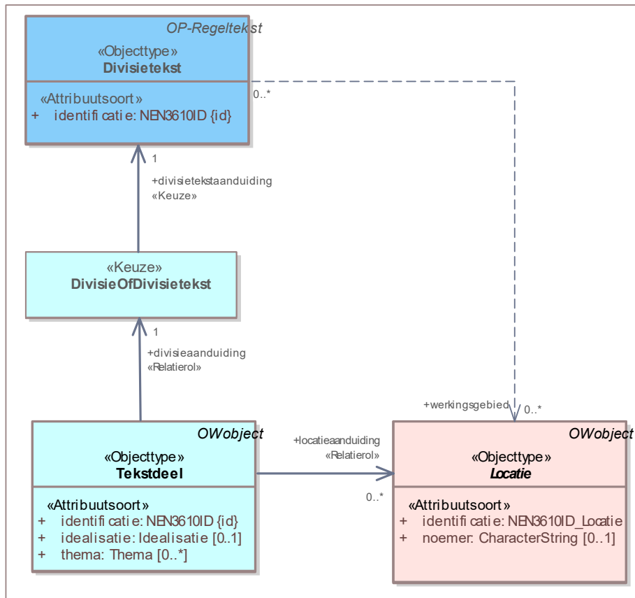
Figuur 29 Uitsnede uit IMOW-diagram voor objecttype Divisietekst
