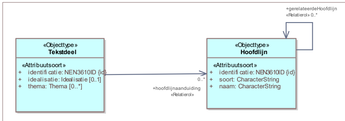
Figuur 31 Uitsnede uit IMOW-diagram voor objecttype Hoofdlijn
